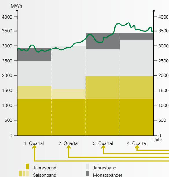
Vertikales Tranchenmodell Erdgas
